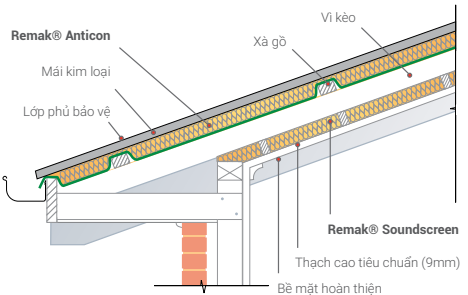
Mẫu 2: Mái kim loại với trần dốc dưới vi kèo
