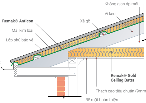
Mẫu 1: Mái kim loại với trần phẳng
